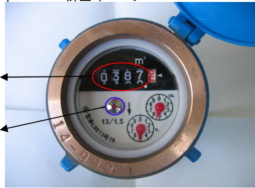
φ13mm新基準メーター
