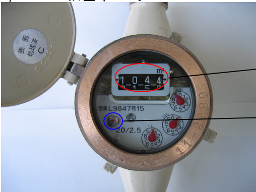
φ20mm旧基準メーター
