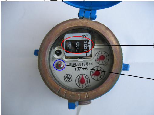
φ13mm旧基準メーター
